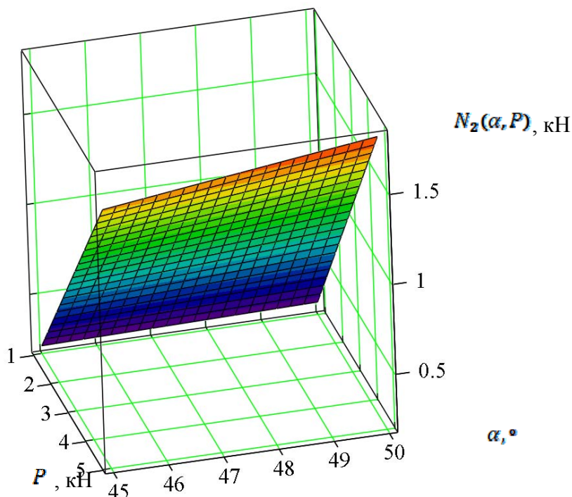
Рисунок 10 – Модель детермінованого факторного аналізу для N_2(\alpha, P) в режимі розвантаження енергетичного засобу та навантаження борони Джерело: розроблено авторами
