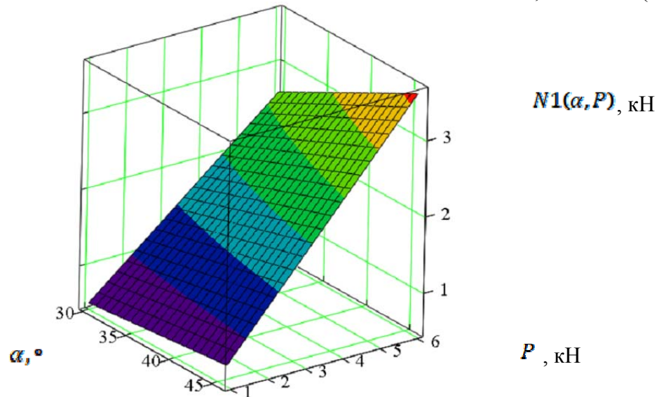
Рисунок 6 – Модель детермінованого факторного аналізу для N_1 в режимі навантаження енергетичного засобу та розвантаження борони
