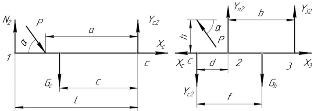
Рисунок 9 – Розрахункова схема до рівняння рівноваги снічі та рами борони МТА (компенсатор зчіпної ваги в режимі розвантаження енергетичного засобу та навантаження борони)
